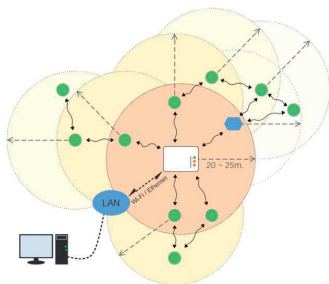
Figur 1: Eksempel på nettverksoppsett
