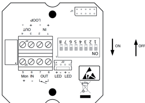
Enkel overvåket inngangsenhet BN-303
